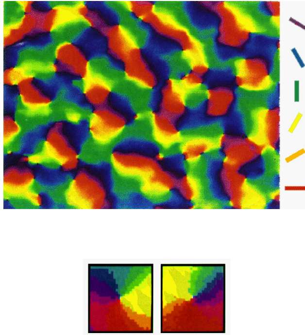
Abbildung 2.6: Oben: Karte der Orientierungspräferenz aus dem primären visuellen Cortex eines Makaken (aus BLASDEL, 1992b). Unten: Beispiel für Pinwheels mit Chiralität (2.1) q_i = +\frac{1}{2} (links) und q_i = -\frac{1}{2} (rechts). Die Orientierung ändert sich beim linken Pinwheel im Uhrzeigersinn von gelb nach rot (d.h. von rechts oblique nach horizontal); beim rechten Pinwheel verläuft die Orientierungsänderung im Urzeigersinn von rot nach gelb (d.h. von horizontal nach rechts oblique; aus BONHOEFFER und GRINVALD, 1991).
