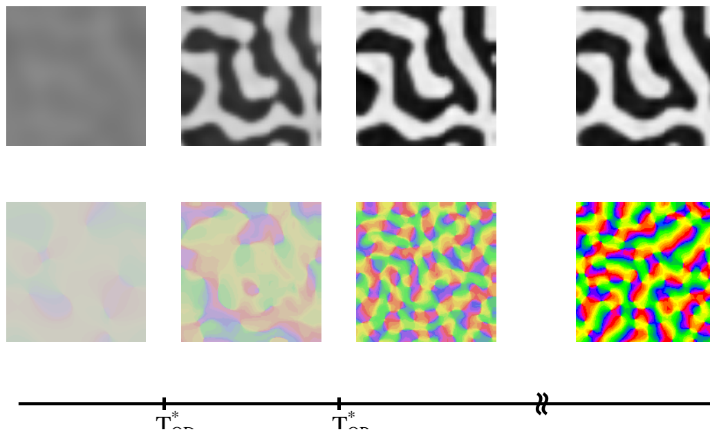
Abbildung 4.5: Momentaufnahmen wie oben, jedoch in einer Simulation mit \sigma_{OD}^* > \sigma_{OP}^* , entsprechend des Szenariums in Abb. 4.1b ( 40 \times 40 Neurone mit periodischen Randbedingungen, \eta_{rel} = 0.0025 , \sigma_{OD}^* = 0.0976 , \sigma_{OP}^* = 0.0679 \implies \Lambda_{OD}/\Lambda_{OP} = 6/5 ).
