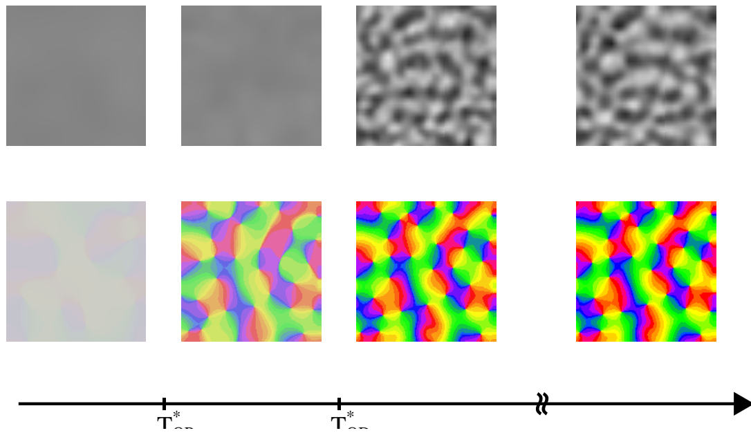
Abbildung 4.4: Momentaufnahmen der koordinierten Entwicklung von Okulardominanz- und Orientierungskarten für \sigma_{OP}^* > \sigma_{OD}^* (Szenarium Abb. 4.1a). Die Farb- / Grauwertintensität spiegelt die Amplitude der Strukturen wieder ( 40 \times 40 Neurone mit periodischen Randbedingungen, \eta_{rel} = 0.0025 , \sigma_{OD}^* = 0.0837 , \sigma_{OP}^* = 0.1189 \implies \Lambda_{OD}/\Lambda_{OP} = 4/5 ).
