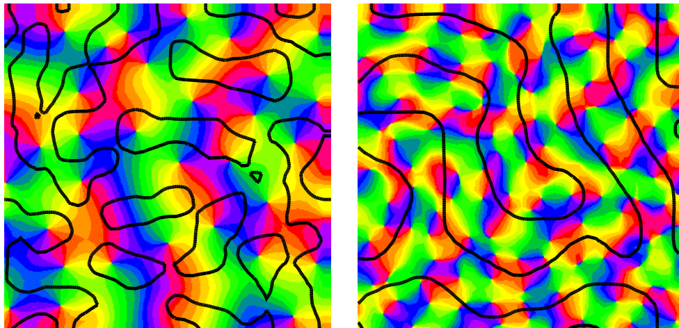
Abbildung 4.6: Vorhersage des funktionalen Layouts von Okulardominanz- und Orientierungspräferenz-Karten für die Katze (links, Ergebnis der in Abb. 4.4 gezeigten Simulation) und den Affen (rechts, Ergebnis der in Abb. 4.5 gezeigten Simulation). Die Abbildungen zeigen eine Überlagerung der Iso-Orientierungsdomänen (farbig) mit den Grenzlinien der Okulardominanzkolumnen (schwarz).
