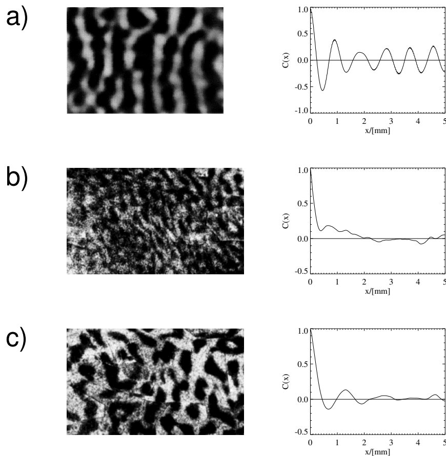
Abbildung 4.2: Die Bilder zeigen typische Auschnitte des OD-Musters aus V1 eines Affen (6.4mm×4.3mm, optisches Ableiten, GRINVALD u. a., 1991) und aus A17 einer normalsichtigen und strabismischen Katze (jeweils 5mm×3mm, ^3\text{H} -Prolin Markierung, LÖWEL und SINGER, 1987). Neben jedem Bild ist die dazugehörige Autokorrelation C(\mathbf{r})|_{\mathbf{r}=\begin{pmatrix} x \\ 0 \end{pmatrix}} gezeigt.
