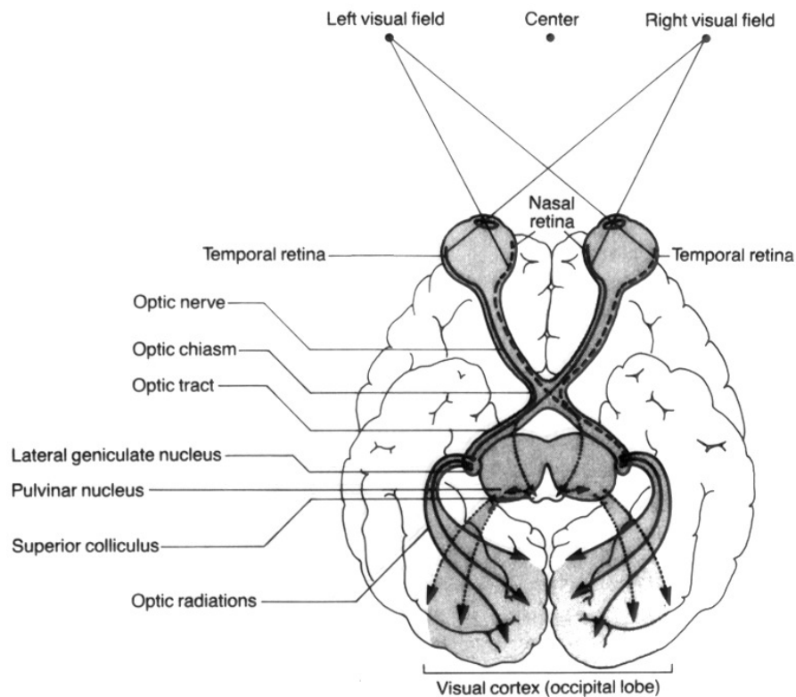
Abbildung 2.1: Skizze der Sehbahn im menschlichen Gehirn von den Augen bis zum primären visuellen Cortex (aus CHURCHLAND und SEJNOWSKI, 1992).
