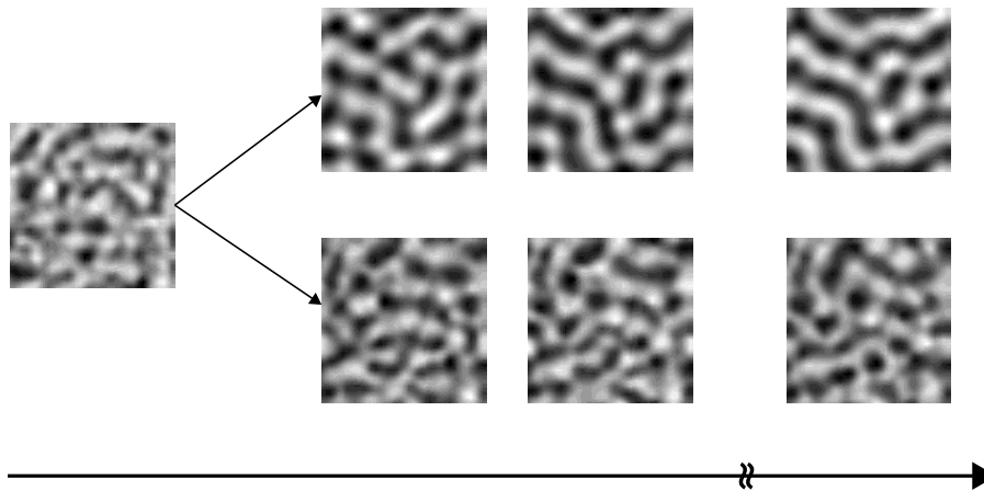
Abbildung 4.7: Momentaufnahmen der Weiterentwicklung einer Okular Dominanzkarte. Die am Anfang gezeigte Karte entstand in einer typischen Simulation mit \sigma_{OP}^* > \sigma_{OD}^* . Ihre Weiterentwicklung in dieser Simulation zeigt die untere Reihe. Die obere Reihe zeigt die Weiterentwicklung der Karte ohne das Muster der Orientierungspräferenz (beide Reihen: 40 \times 40 Neurone, \sigma(t) = \sigma_{OD}^* * 0.9 , \eta_{rel} = 0.001 ).
