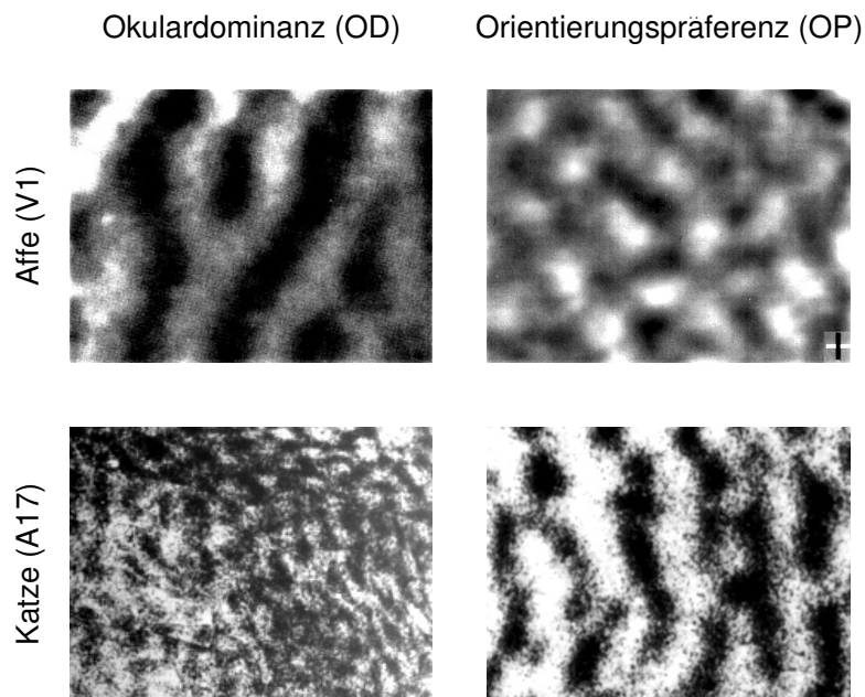
Abbildung 2.7: Layoutvergleich kolumnärer Strukturen aus dem primären visuellen Cortex von Katzen (Daten aus LÖWEL und SINGER, 1987; LÖWEL und SINGER, 1990) und Affen (Daten aus BLASDEL, 1992a).
