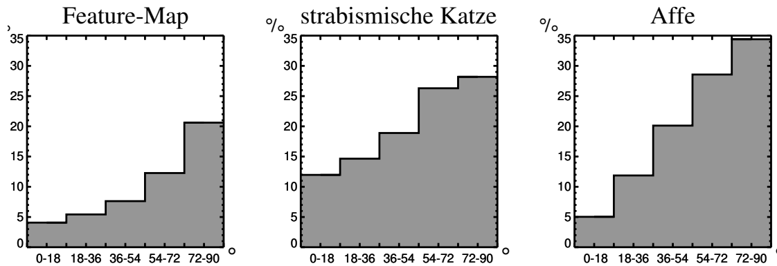
Abbildung 2.11: Histogramme der Schnittwinkelverteilung zwischen den Iso-Orientierungslinien und den Grenzlinien der Okulardominanzdomänen im phänomenologischen Modell (siehe Abschn. 3), der strabismischen Katze (hier für den in Abb. 2.10 gezeigten Datensatz; weitere siehe LÖWEL u. a., 1996) und den Affen (Daten aus OBERMAYER und BLASDEL, 1993).
