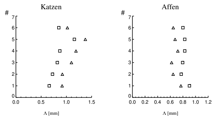
Abbildung 2.7: Layoutvergleich kolumnärer Strukturen aus dem primären visuellen Cortex von Katzen (Daten aus LÖWEL und SINGER, 1987; LÖWEL und SINGER, 1990) und Affen (Daten aus BLASDEL, 1992a).
