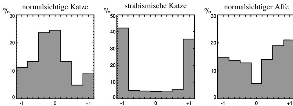
Abbildung 2.9: Okulardominanzhistogramme für normalsichtige und strabismische Katzen, sowie für den Affen. Es ist die relative Häufigkeit der Zellen, die sich entweder nur vom linken (-1) oder nur vom rechten (+1) oder von beiden Augen (0) stimulieren lassen aufgetragen. Bei normalsichtigen Katzen sind die meisten Zellen binokular. Bei strabismischen Katzen und beim Affen überwiegt die Zahl der Zellen, die sich auf eines der beiden Augen spezialisiert hat (Daten aus HUBEL, 1989).
