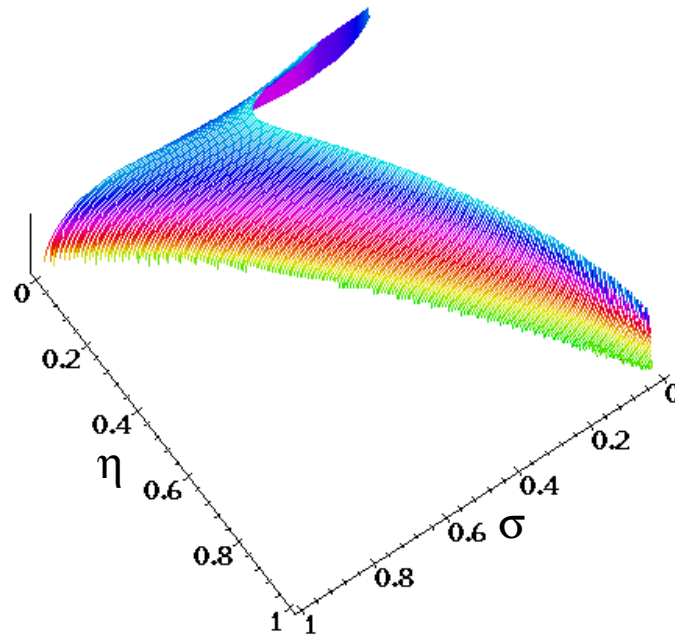
Abbildung 3.3: Amplitude (3.9) des Lösungsansatzes (3.8) gezeigt für A \in [0 \dots 0.7] (zur besseren Übersicht farbig kodiert).
