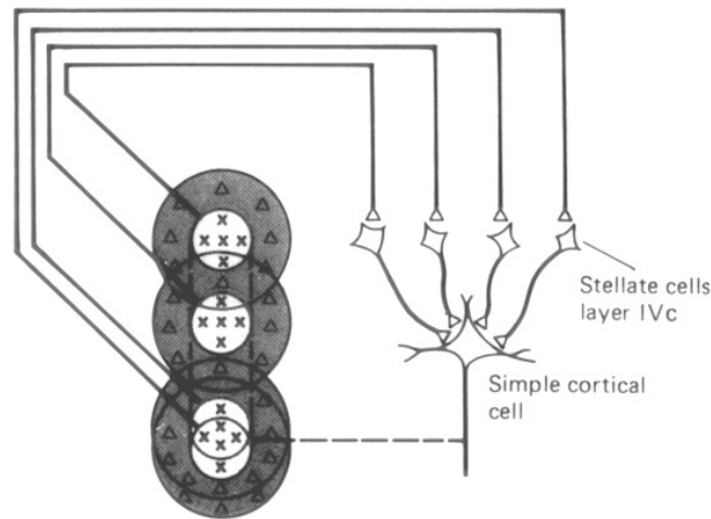
Abbildung 2.3: Einfaches Model der Orientierungspräferenz HUBEL und WIESEL, 1962: Die Axone mehrerer Zentrum–Umfeld–Zellen konvergieren auf eine einfache Zelle. Dadurch, daß die rezeptiven Felder der Zentrum–Umfeld–Zellen auf der Sinnesoberfläche entlang einer Linie angeordnet sind, antwortet die einfache Zelle selektiv auf Lichtbalken einer bestimmten Orientierung.
